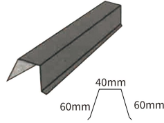
Square Ridge Cap 方型脊瓦
