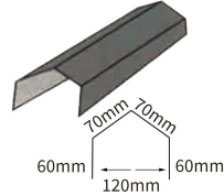
Angle Ridge Cap I 角型脊瓦1
