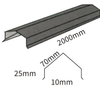
Angle Ridge Cap II 角型脊瓦2
