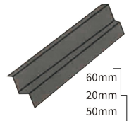
Wall Side Flashing 泛水板
